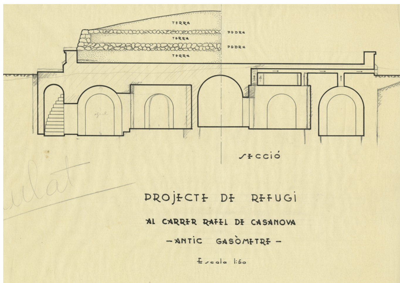
Projecte de refugi del carrer Gasòmetre de Tarragona, 1937, 74 cm [Plànols d'Arquitectura, capsa 67]
