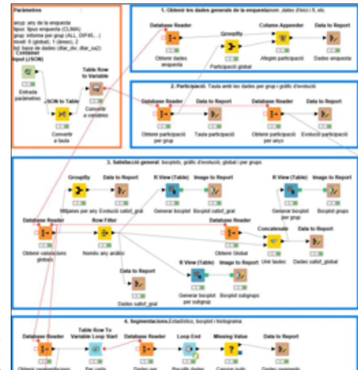
Captura de pantalla de l'eina Knime on es pot veure parcialment el flux d'anàlisi de les dades.
