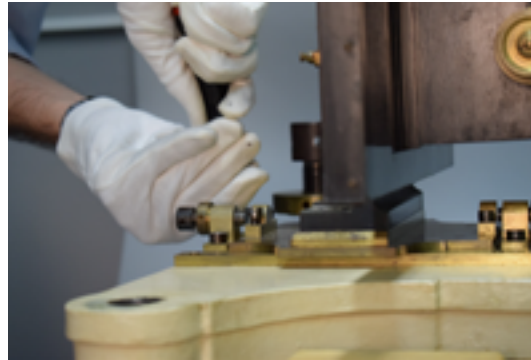
Espectroheliògraf tipus Evershed. Observatori de l'Ebre.
