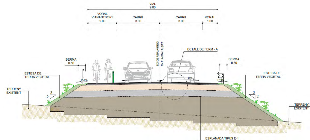
Figura 1. Secció tipus d'un tram de variant
